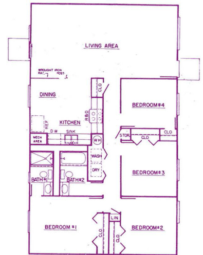
Plan 632
